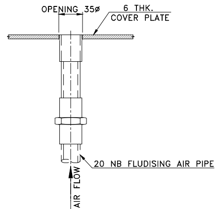
DETAIL Y
